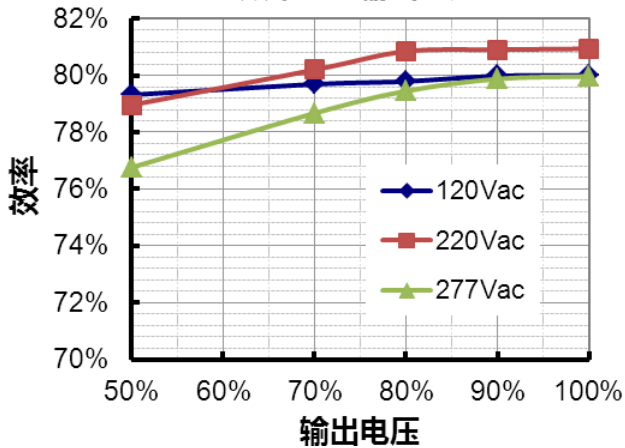
LUC-012S070DSM(SSM) 效率 vs. 输出电压
