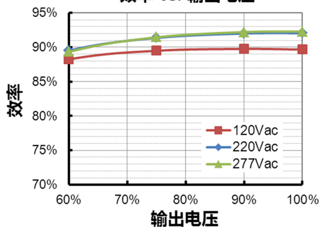
EUP-096S215ST( I_o=1750mA )
