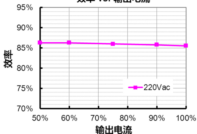
EBV-100S012SV 效率 vs. 输出电流
