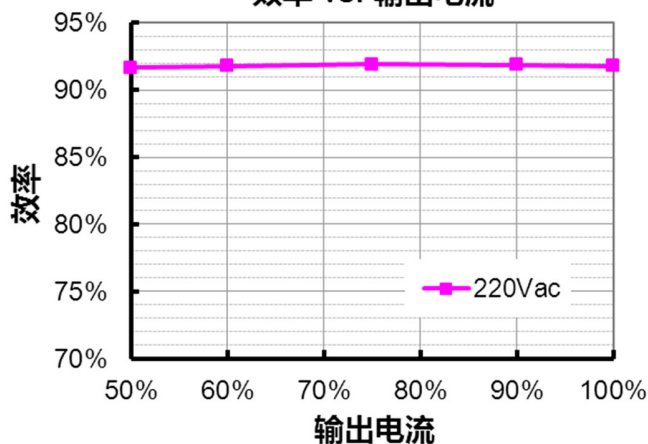
EBV-100S048SV 效率 vs. 输出电流
