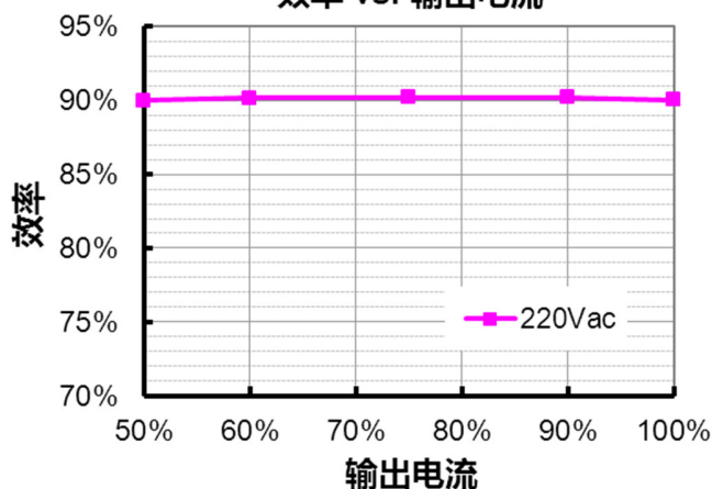
EBV-100S024SV 效率 vs. 输出电流
