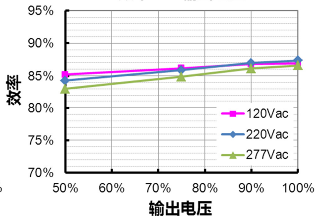
EUC-026S070SVM (I o =700mA) 效率 vs. 输出电压
