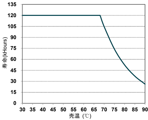
寿命对壳温曲线
