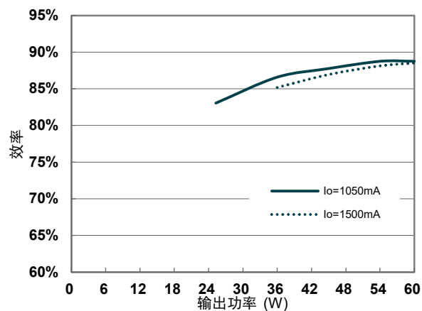
效率@220Vac
