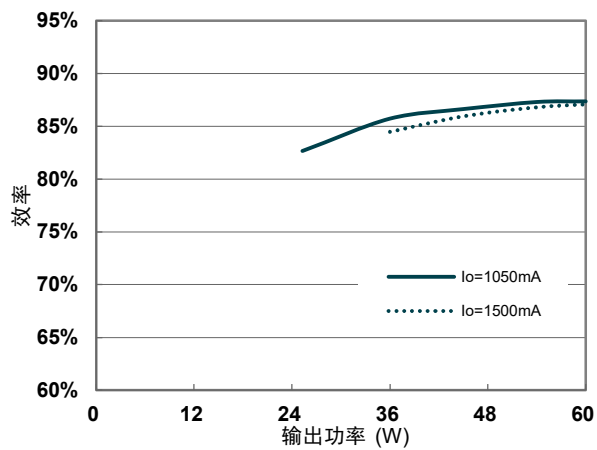
效率@220Vac
