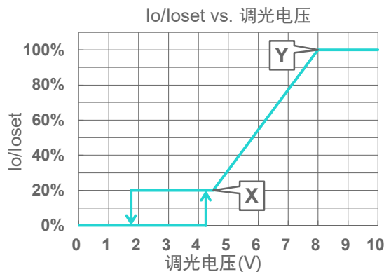
示意图 7：正逻辑
