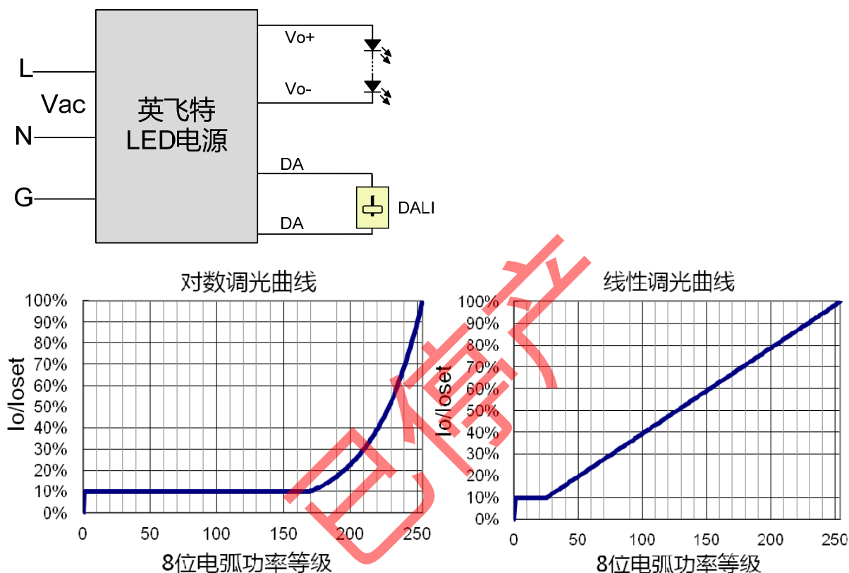
示意图: DALI 调光
