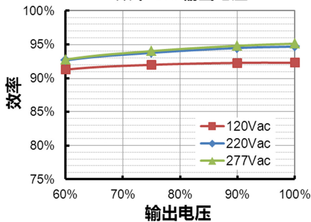
EUD-600S560DV( I_o=4480mA ) 效率 vs. 输出电压
