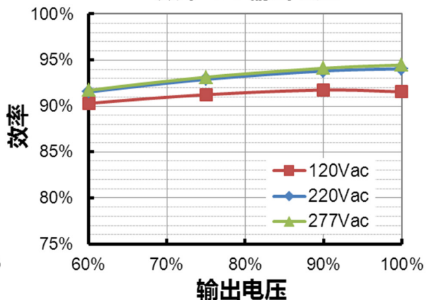
EUD-600S560DV( I_o=5600mA ) 效率 vs. 输出电压
