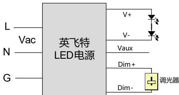
示意图 3: 正逻辑
