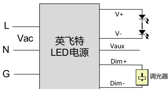
示意图 4: 负逻辑
