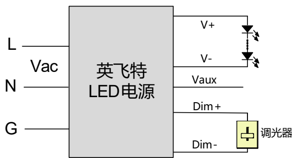
示意图 2: 负逻辑
