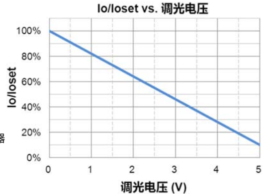
示意图 2: 负逻辑
