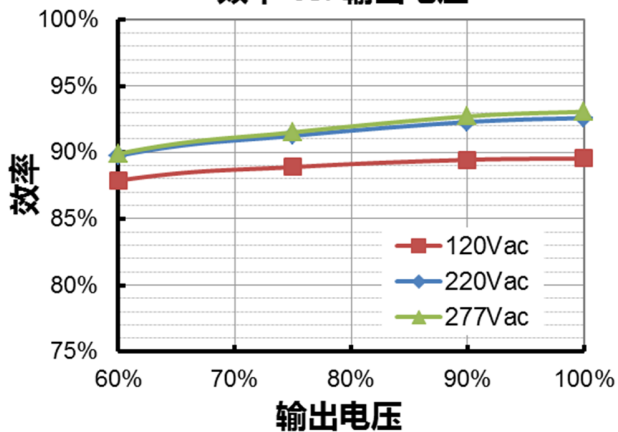
EUK-240S420DV(TV)( I_o=2800mA ) 效率 vs. 输出电压
