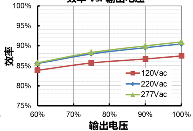
EUK-240S420DV(TV)( I_o=4200mA ) 效率 vs. 输出电压
