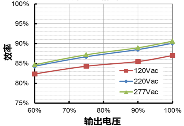
EUK-240S670DV(TV)( I_o=6700mA ) 效率 vs. 输出电压
