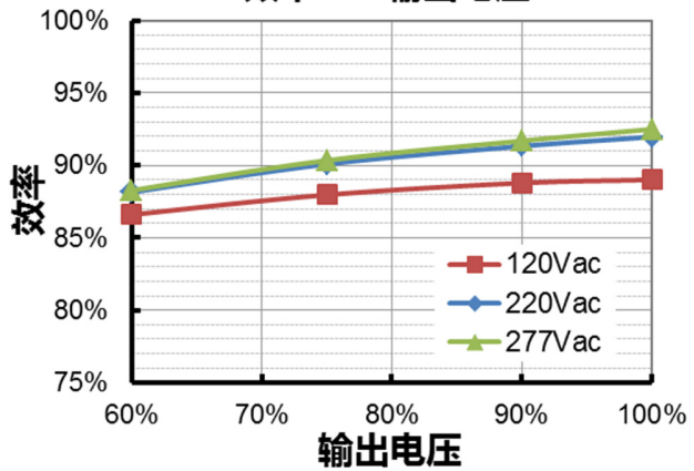
EUK-240S210DV(TV)( I_o=2100mA ) 效率 vs. 输出电压
