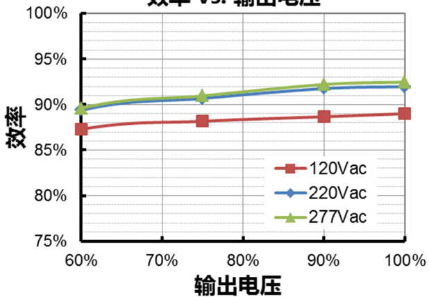
EUK-240S670DV(TV)( I_o=4600mA ) 效率 vs. 输出电压
