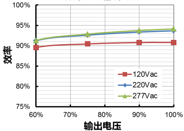
EUK-240S210DV(TV)( I_o=1400mA ) 效率 vs. 输出电压
