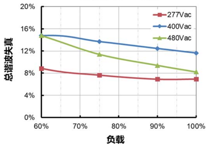
总谐波失真 vs. 负载
