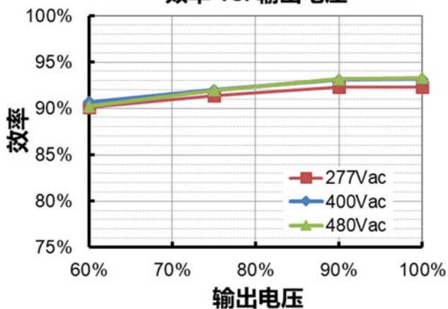
ESM-150S150Mx( I_o=1050mA ) 效率 vs. 输出电压
