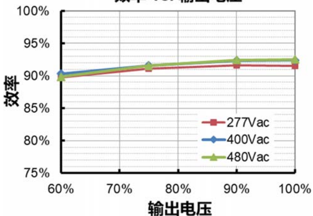
ESM-150S210Mx( I_o=1400mA ) 效率 vs. 输出电压
