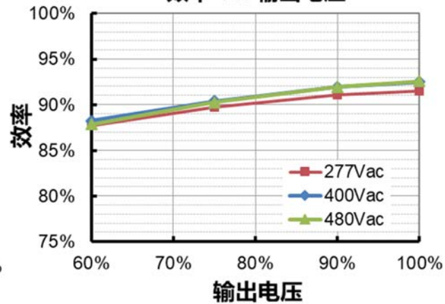
ESM-150S210Mx( I_o=2100mA ) 效率 vs. 输出电压
