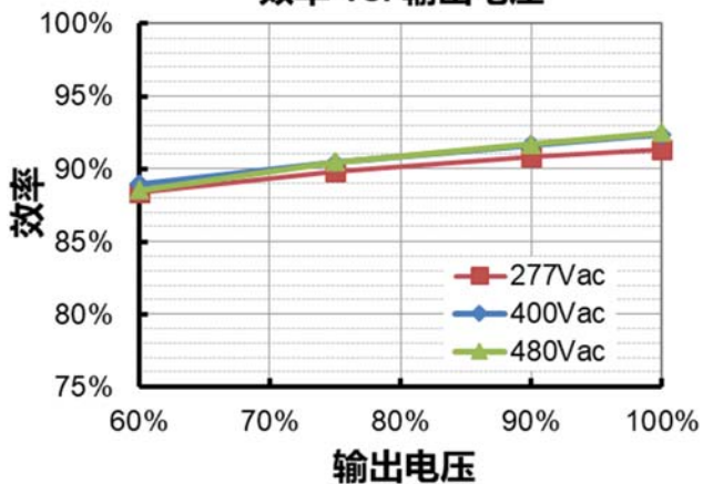
ESM-150S150Mx( I_o=1500mA ) 效率 vs. 输出电压
