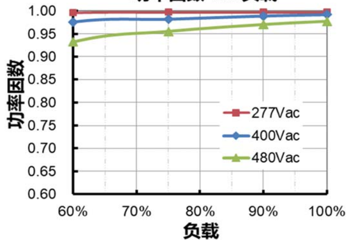
功率因数 vs. 负载
