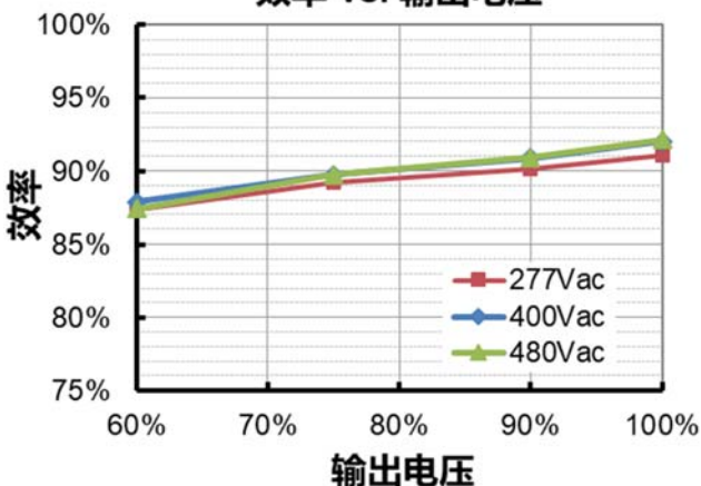
ESM-150S210Mx( I_o=2100mA ) 效率 vs. 输出电压
