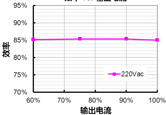
EBV-048S048SVF 效率 vs. 输出电流
