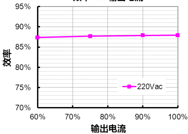
EBV-048S048SVF 效率 vs. 输出电流
